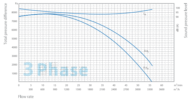
MAb-55C/T
