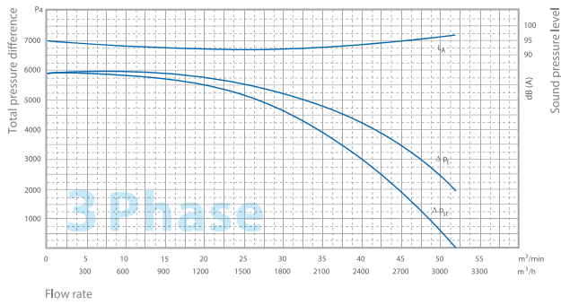
MAb-55B/T
