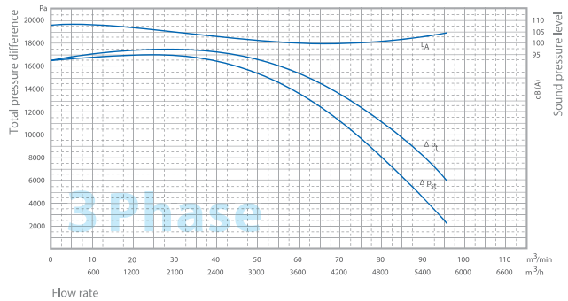
MAb-60C/T
