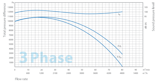
MAb-60A/T
